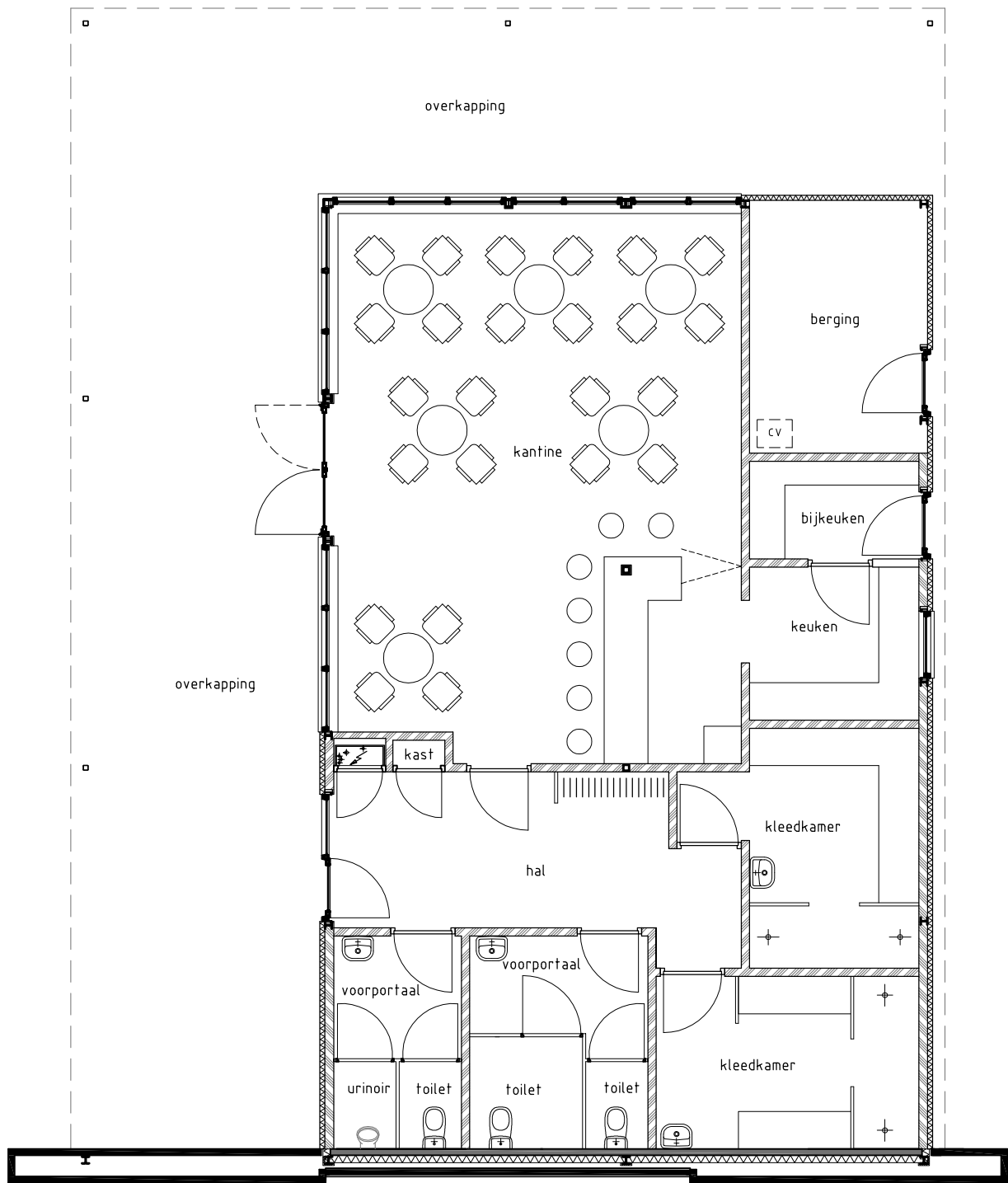
plattgrond
